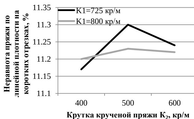
Рисунок 3 – Влияние крутки одиночной и крученой пряди на неравноготу по линейной плотности крученой пряди
