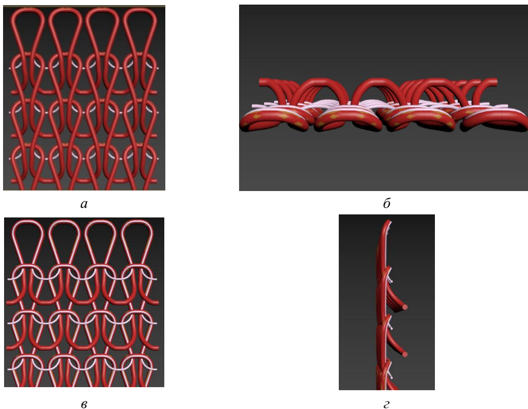
Рисунок 2 – Готовая 3D-модель трикотажа плюшевого переплетения: а – лицевая сторона; б – изнаночная сторона; в – вид сверху; г – вид сбоку
