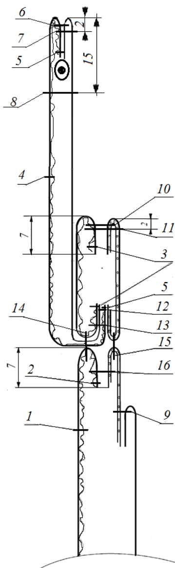
Рисунок 3 – Обработка капюшона и соединение его с горловиной изделия
