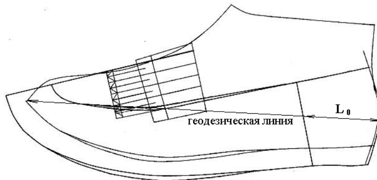
Рисунок 1 – Схема замера длинотных параметров деталей заготовки
