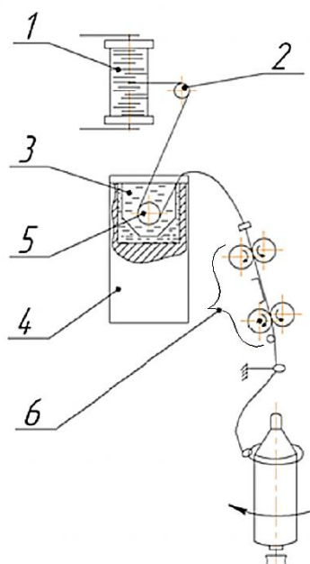
Рисунок 1 – Технологическая схема прядильной машины ПМ-88-Л5 с ультразвуковой установкой
