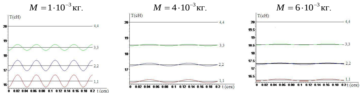
Рисунок 2 – Изменение натяжения по времени в различных углах \varphi дуги контакта при относительной скорости пряжи v = 30 \text{ м/мин} и различных значениях массы воронки M
