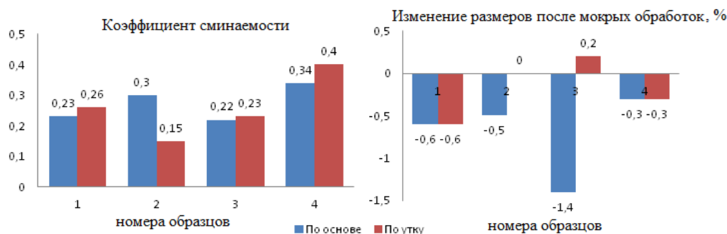
Рисунок 2 – Результаты исследования сминаемости и изменения размеров после мокрых обработок льносодержащих костюмных тканей по основе и утку
