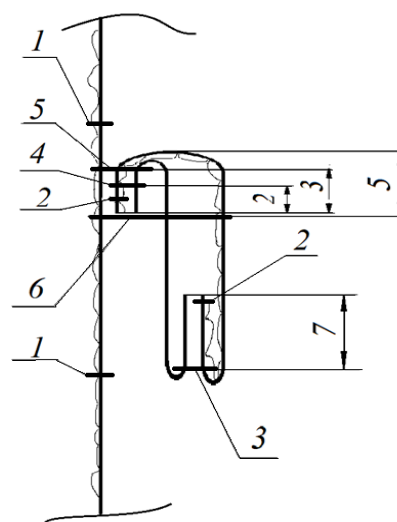
Рисунок 2 – Обработка края борта
