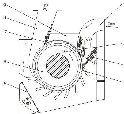
Рисунок 4 – Волоконоочиститель с измененным углом подачи по патенту Узбекистан, № FAP00829: 1 – вход волокна; 2 – пильный цилиндр; 3 – щетка; 4 – колосниковая решетка; 5 – жалюзи; 6 – прокладка; 7 – нож; 8 – выход волокна; 9 – щит
