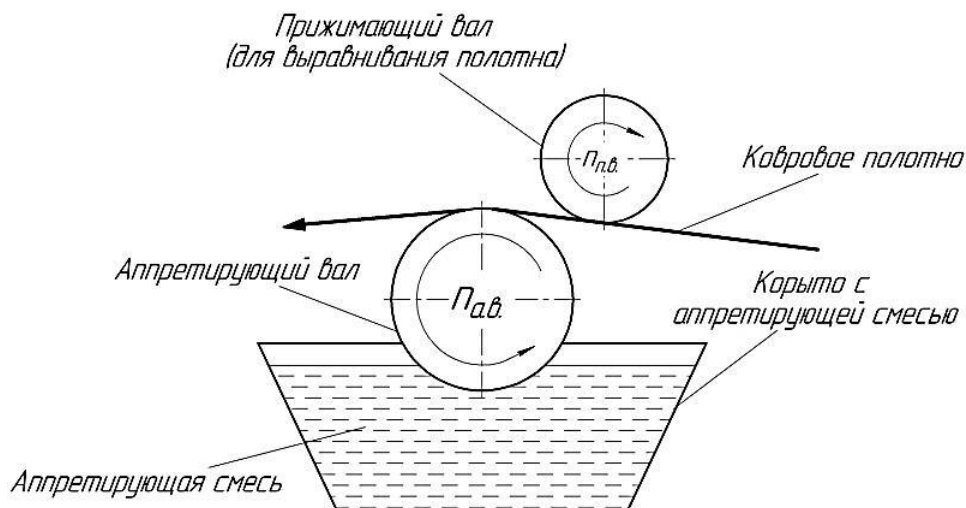
Рисунок 1 – Схема нанесения аппретирующей смеси на изнаночную сторону коврового покрытия на аппретурной машине Bajimac-SA
