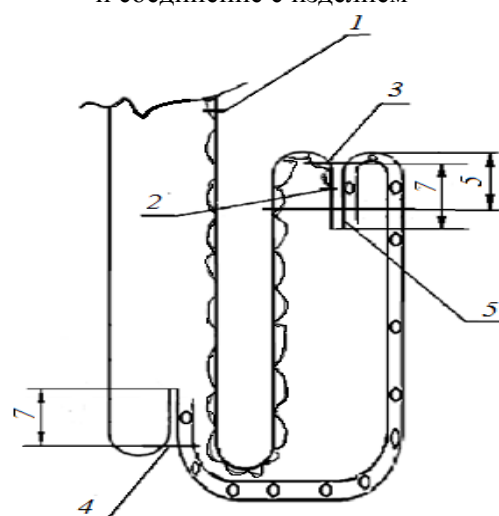
Рисунок 4 – Обработка клапана и соединение с изделием
