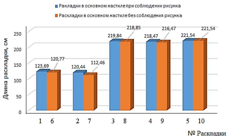
Рисунок 3 – Длина раскладок при различных вариантах сочетаний
