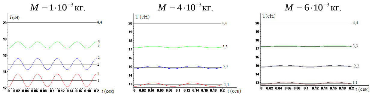
Рисунок 1 – Изменение натяжения по времени в различных углах \varphi дуги контакта при относительной скорости пряжи v = 10 \text{ м/мин} и различных значениях массы воронки M
