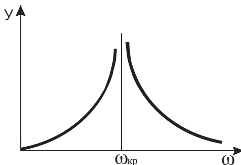
Рисунок 2 – Зависимость прогиба пыльного цилиндра от его угловой скорости вращения
