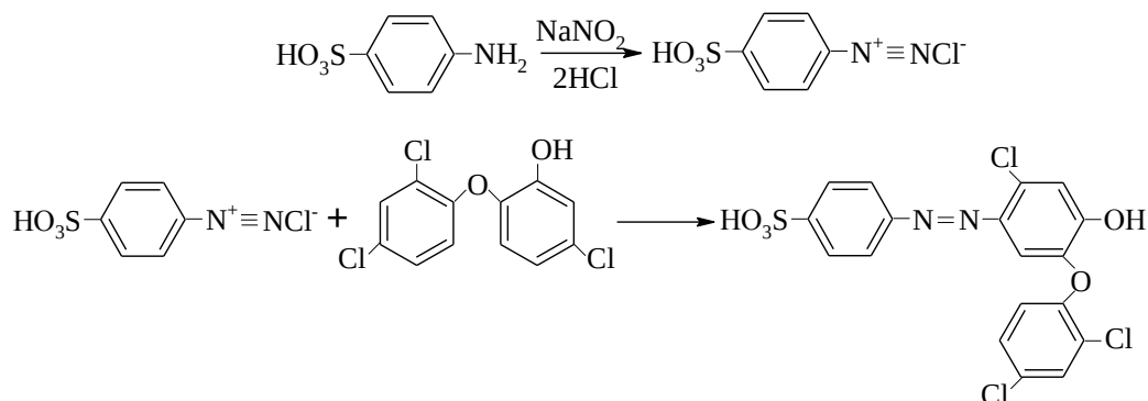
Рисунок 2 – Схема синтеза красителя на основе сульфаниловой кислоты и триклозана
