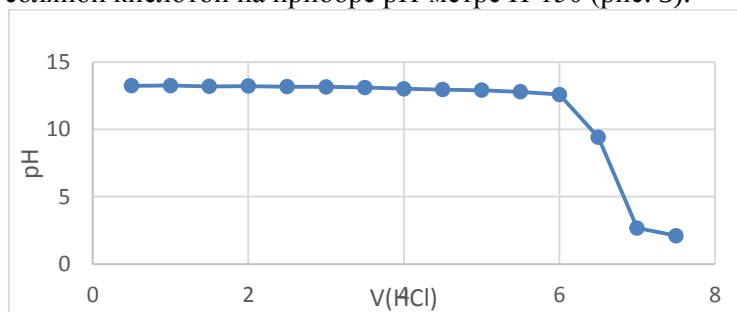
Рисунок 3 – Зависимость pH среды красителя на основе сульфаниловой кислоты от объема (см³) 2Н соляной кислоты
