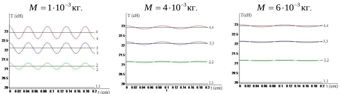
Рисунок 3 – Изменение натяжения по времени в различных углах \varphi дуги контакта при относительной скорости пряжи v = 50 \text{ м/мин} и различных значениях массы воронки M
