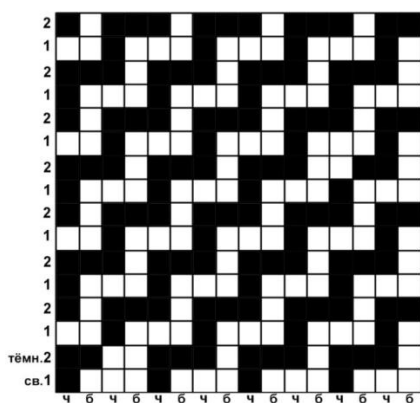
Модельное переплетение для красных участков
