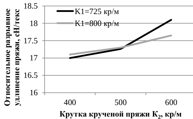
Рисунок 2 – Влияние крутки одиночной и крученой арселоновой пряди на относительное разрывное удлинение крученой пряди
