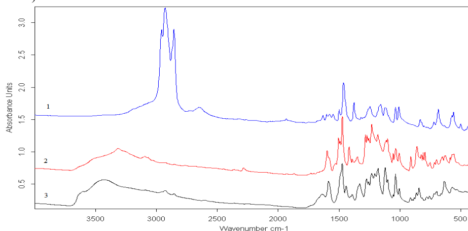
Рисунок 4 – ИК-спектры: 1 – сульфаниловая кислота, 2 – краситель в кислой среде, 3 – краситель в щелочной среде
